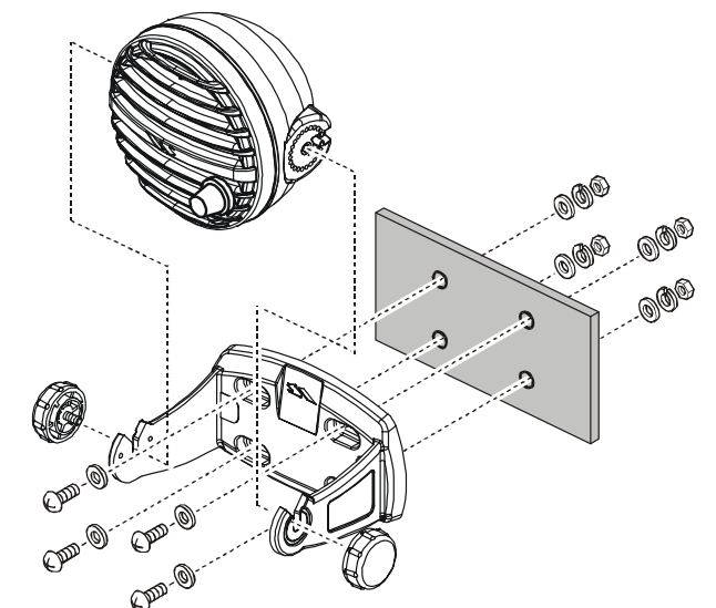
Figure 2 (Wall Mount)
